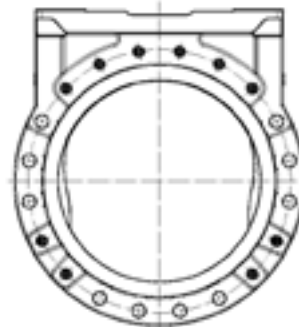
PN 16/10 DN 500–600
