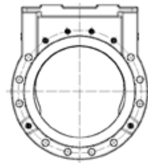
PN 16/10 DN 350–400
